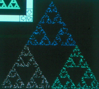
Sierpinski-1500 (Graphic)
