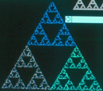
Sierpinski-4500
