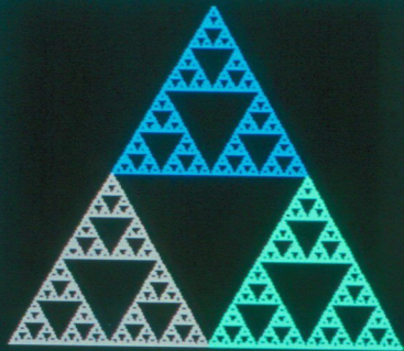
Sierpinski-4500
